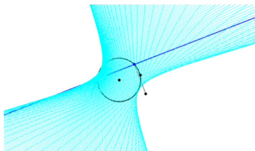
図 4 包絡線としての双曲線
