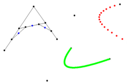
図 6 ベジエ曲線の構成
